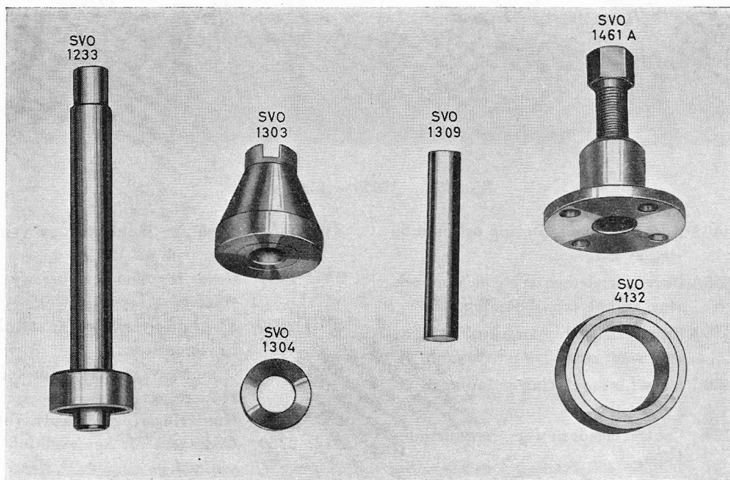
Bild 114. Verktyg för vattenpump av tidigare utförande.
